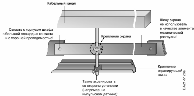
Рис. 5/36 Экранирование при вводе в шкаф.
