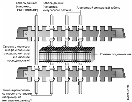
Рис. 5/37 Экранирование в электрическом шкафу.
