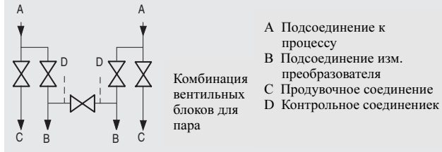
Комбинация вентильных блоков DN 5/DN 8, схема
