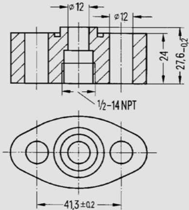
Овальный фланец, размеры в мм
