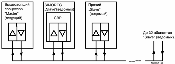
Рис. 4/24 Связи PROFIBUS-DP
