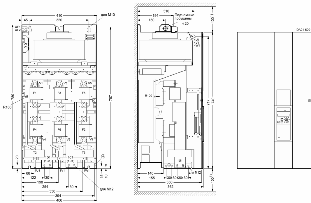
Рис. 8/12 AC 400 V, 575 V, 690 V и 830 V, 1500 A ... 2000 A
